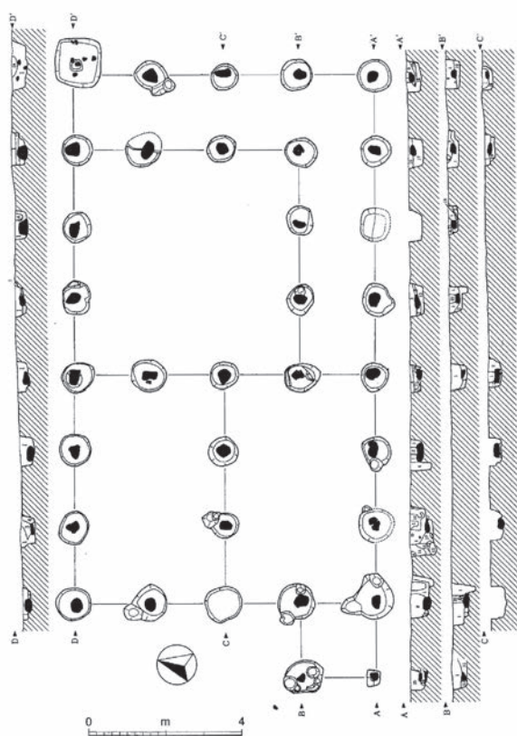
図12 礎盤石柱建物実測図（浪岡町 2002）
