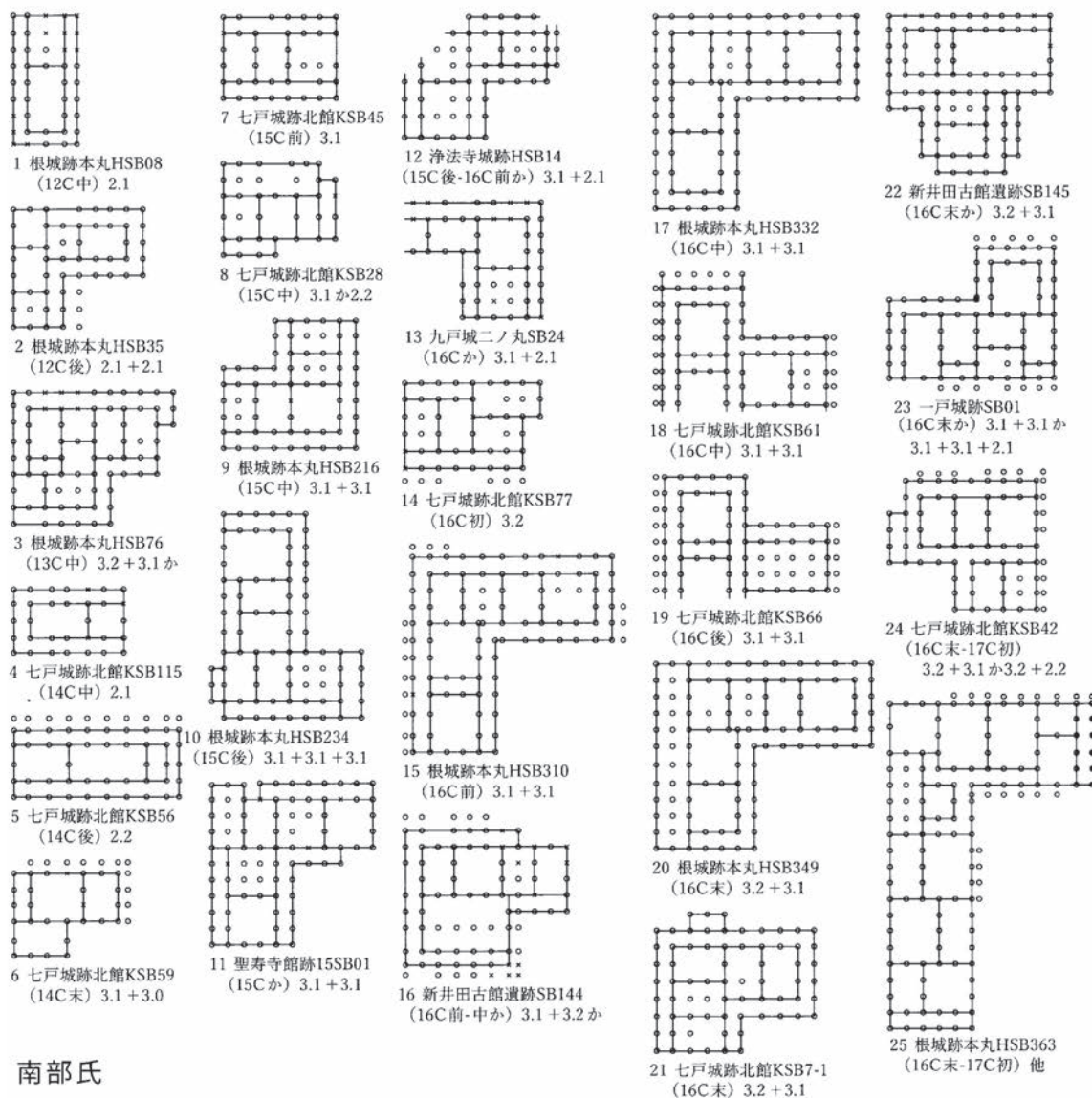
図15 糠部郡で検出された大型建物模式図（中村 2019）
